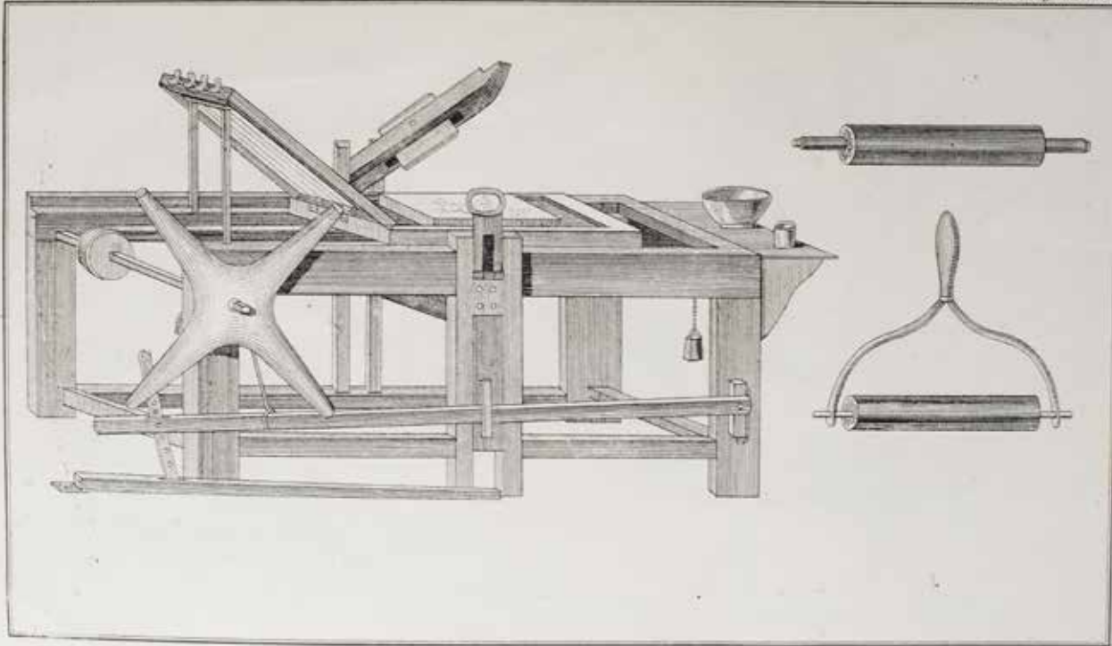
Ständruckpresse mit den Schwarzwalzen.
